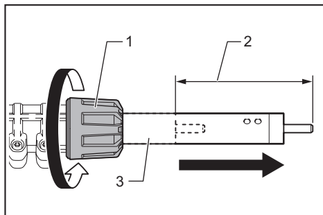
► 1. Anillo de bloqueo 2. 10 cm o más 3. Tubo
