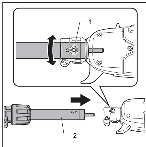
► 1. Agujero 2. Tubo
