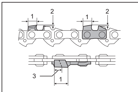
▶ 1. Longitud de la cuchilla 2. Distancia entre el borde cortante y el calibre de profundidad 3. Longitud mínima de la cuchilla (3 mm)
