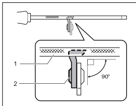
► 1. Lima 2. Cadena de sierra
