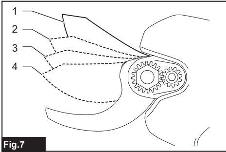
Fig.7 ► 1. ø30 mm 2. ø25 mm 3. ø18 mm 4. ø10 mm
