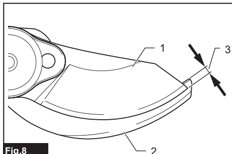
► 1. Cuchilla superior de las tijeras 2. Cuchilla inferior de las tijeras 3. 1 - 3 mm
