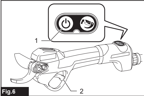
Fig.6 ► 1. Botón de alimentación principal 2. Gatillo interruptor
