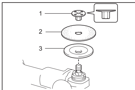
► 1. Contratuercia para lijar 2. Disco abrasivo 3. Plato de caucho
