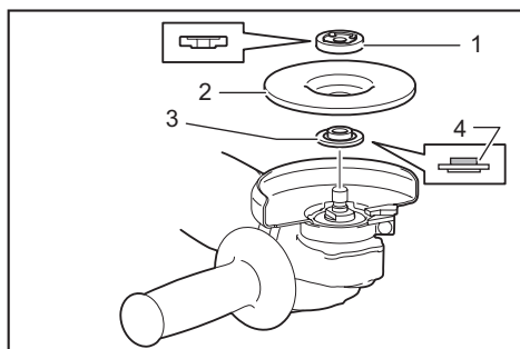
► 1. Contratuercia 2. Muela de centro hundido 3. Brida interior 4. Parte de montaje
