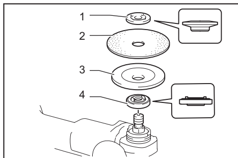
► 1. Contratuercia para lijar 2. Disco abrasivo 3. Plato de caucho 4. Brida interior
