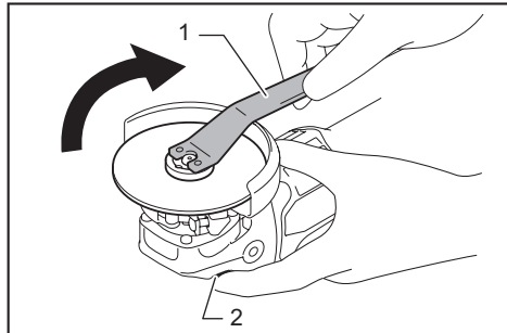
► 1. Llave de contratuercia 2. Bloqueo del eje
