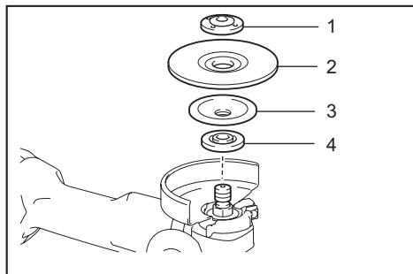
► 1. Contratuercia 2. Disco flexible 3. Plato de respaldo 4. Brida interior
