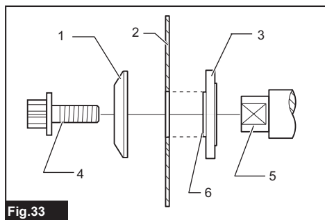
Fig.33 ► 1. Brida exterior 2. Disco 3. Brida interior 4. Perno de cabeza hueca hexagonal (rosca hacia la izquierda) 5. Eje 6. Parte de montaje de disco
