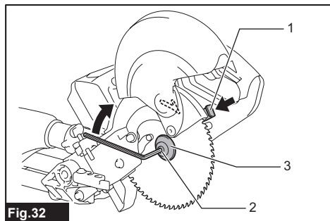
Fig.32 ► 1. Bloqueo del eje 2. Perno de cabeza hueca hexagonal 3. Brida exterior
