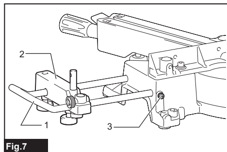
Fig.7 ► 1. Soporte 2. Conjunto de soporte 3. Tornillo
