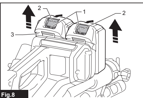
Fig.8 ► 1. Indicador rojo 2. Botón 3. Cartucho de batería
