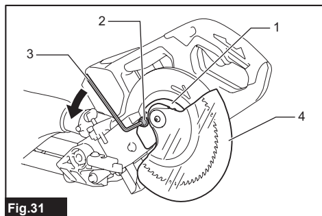
Fig.31 ► 1. Cubierta central 2. Perno de cabeza hueca hexagonal 3. Llave hexagonal 4. Protector de disco
