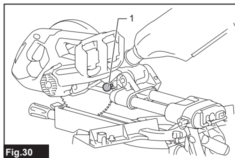
Fig.30 ► 1. Pasador de retención
